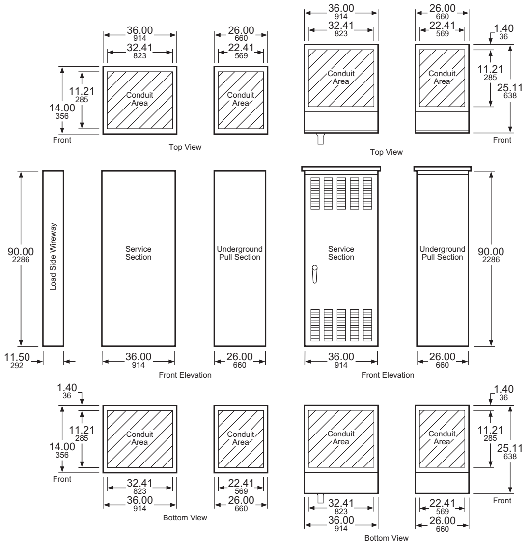
NEMA Type 1
