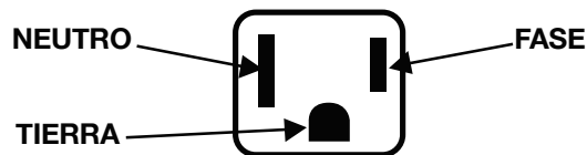
CONFIGURACIÓN DE RECEPTÁCULO NEMA 5-15R
